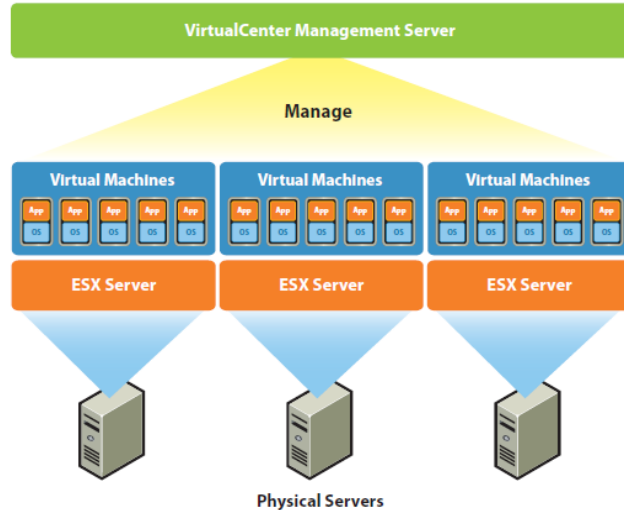
شکل ۱۰-۷- شمای کلی عملکرد سرور VCenter
