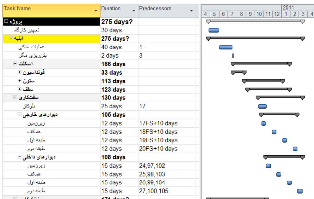
شکل ۱۷-۳۰: تکمیل اطلاعات بلوکاز و دیوارها
